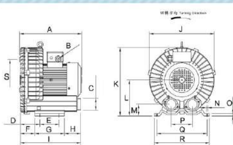
LG-6068 3HP
