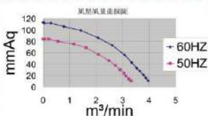
CX-1/4 0.18KW
